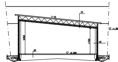
LEIKKAUS KORKEUDET TARKISTETTAVIA VANHAN HALLIN MUKAN
